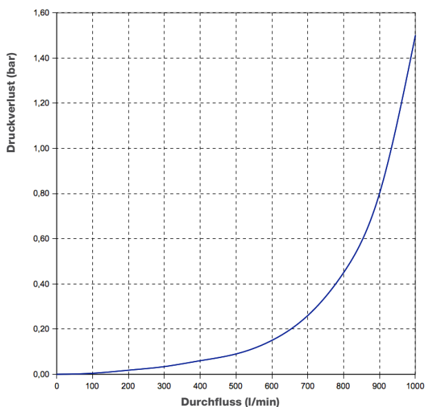
Druckverlust beim Typ AB-F65
